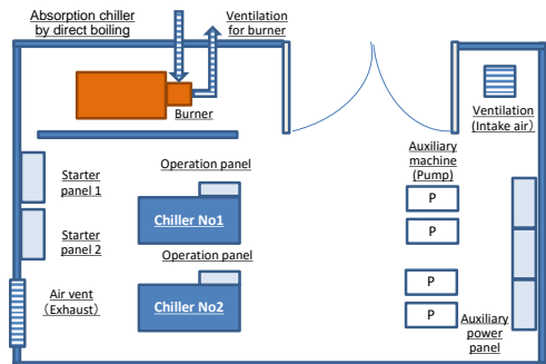
図 9-10 機械室のイメージ
