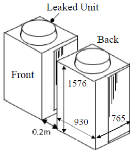
図 8-11 地上設置
