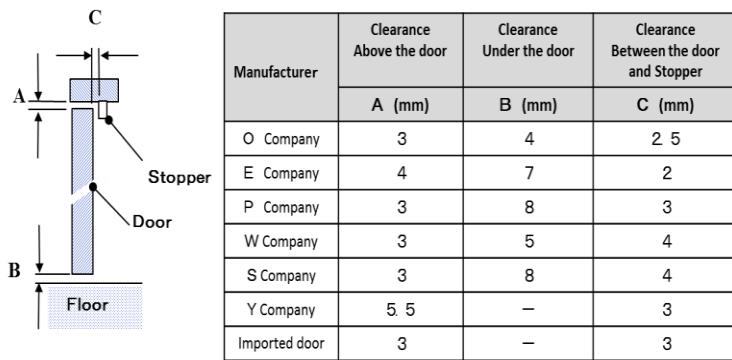
図 6-5 各社の開き戸の隙間寸法
