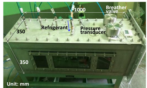
図 3-50 直方体燃焼容器
