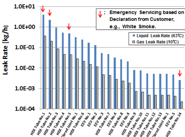
図 8-1 室内機不良部品の漏洩速度
