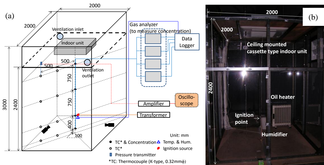
図 3-55 実大着火実験装置全景および燃焼容器写真
