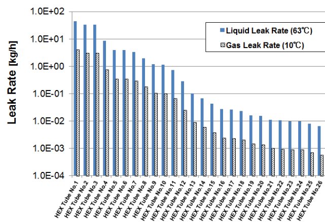
図 8-2 室外機不良部品の漏洩速度
