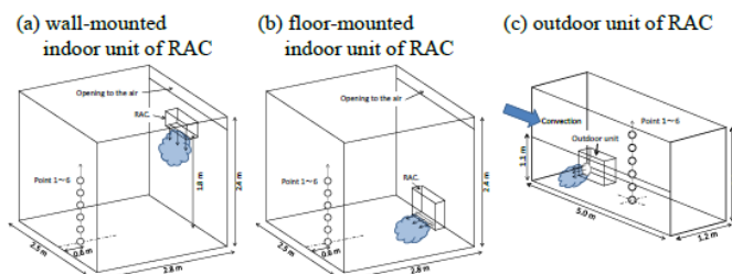
図 6-1 エアコン各機器のシミュレーション状況
