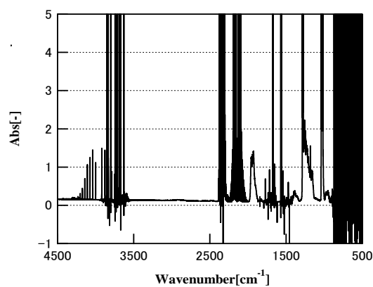
図 3-28 低冷媒濃度時排気ガス吸光スペクトル
