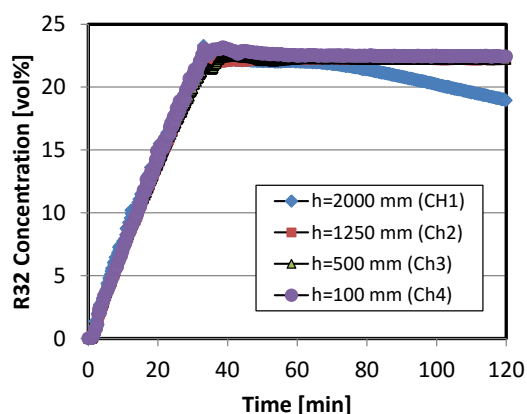
図 3-56 燃焼容器内の R32 濃度の経時変化
