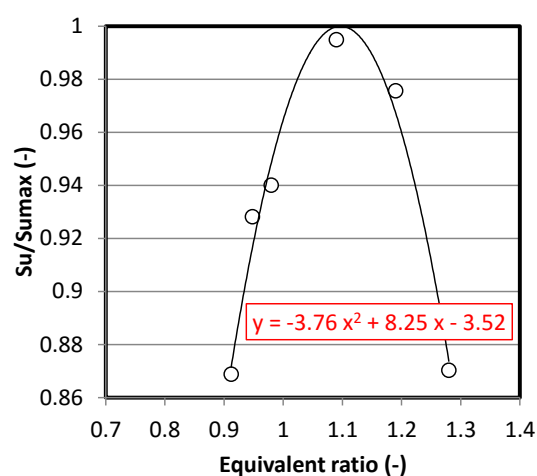
図 3-53 R32 当量比と Su/Su_{max} の関係
