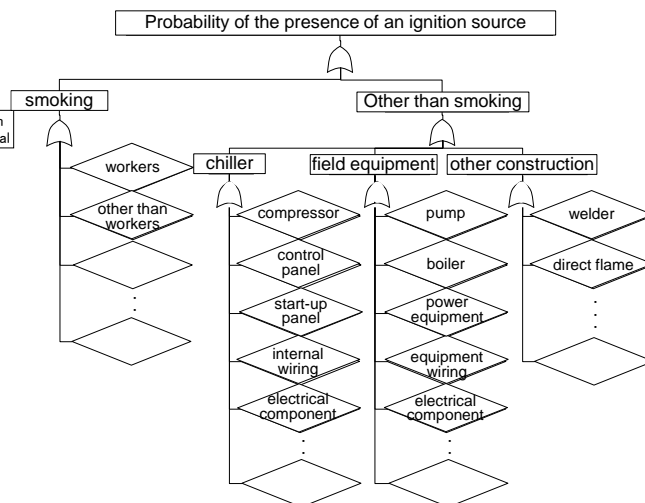
図 9-2 各 LS での着火源評価の標準 FTA
