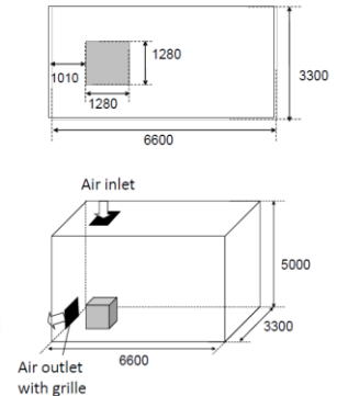
図 8-14 機械室設置
