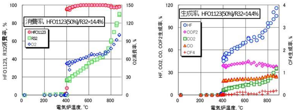
図 2-33 HFO1123/R32 混合冷媒の熱分解. HFO1123(50%)/R32=14.4vol% ( \phi=1.0 ), 冷媒 + 空気流量=100cm 3 /min.
