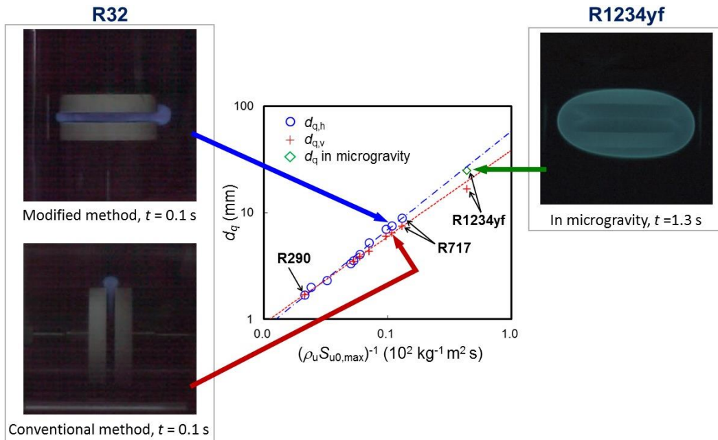
図 2-13 11 化合物の消炎距離 (25°C, 0%RH)
