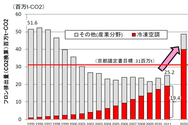
図 1-3 日本冷凍空調分野のフロン排出量
