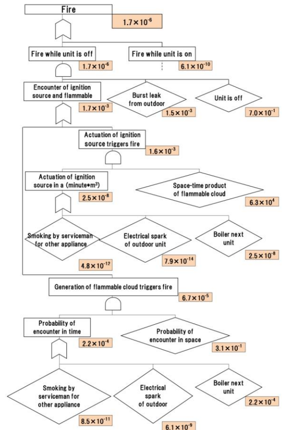
図 8-24 半地下に設置された室外機の使用時 FTA (対策なし)
